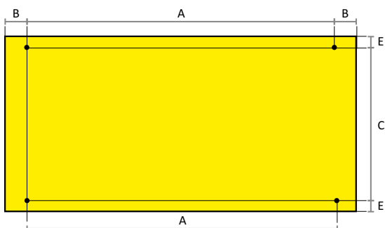
D-FB3 19-xxx asennusreiät - M6 kierre
