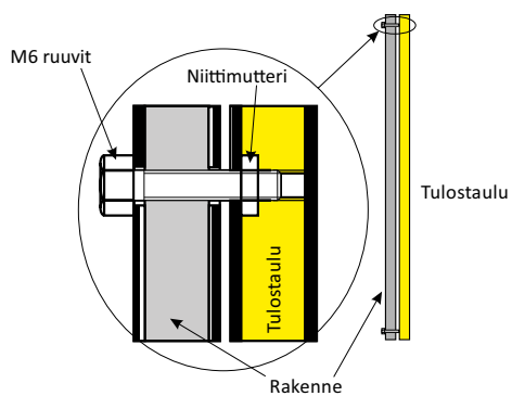
Asennus kehikoon, kiristys M6-pulteilla taulun takaa from the back
